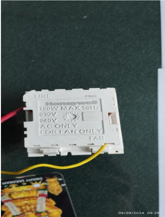
Item no .1 Honeywell Fan Regulator
